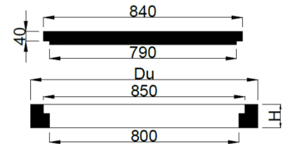
Dæksel Ø800 mm Dækslet består af en topring med fals og et dæksel
