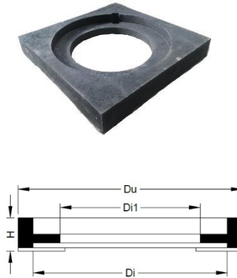
Firkantkarm til Ø315 mm dæksel
