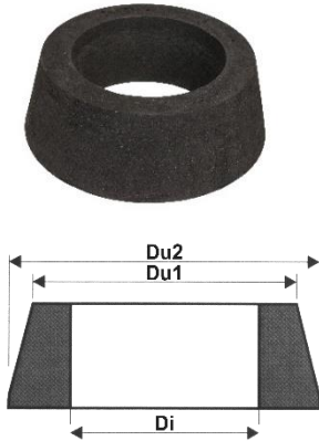
Kegle Ø600 mm
