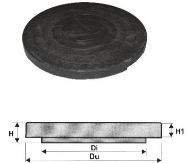
Dæksel Ø800 mm Dækslet består af en topring med fals og et dæksel
