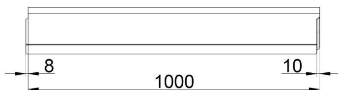
TOP 100 rendeelement
