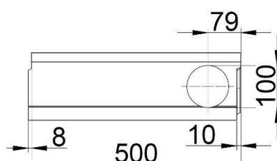
TOP 100 X-rendeelement
