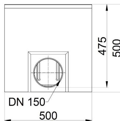
TOP 100 udløbskasse
