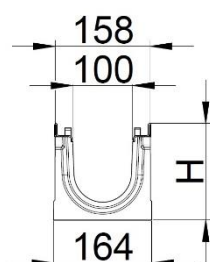
TOP 100 rendeelement
