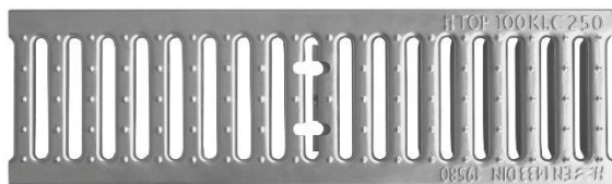
Galvaniseret spalterist Indløbsareal: 359 cm 2 /m
