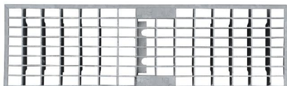
Galvaniseret maskerist 30/10 Indløbsareal: 900 cm 2 /m
