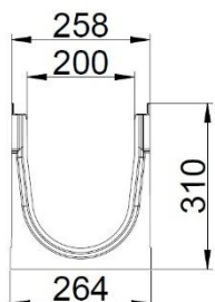
TOP 200 rendeelement
