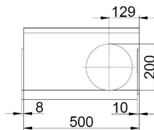
TOP 200 X-rendeelement
