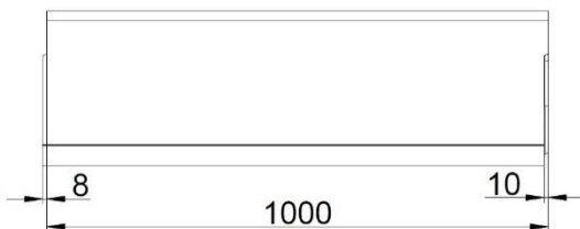
TOP 200 rendeelement
