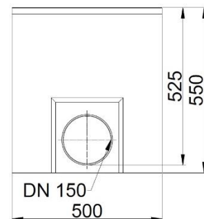
TOP 200 udløbskasse
