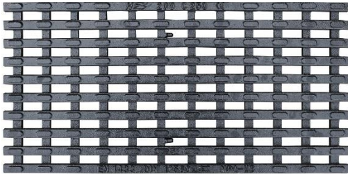
Støbejernsrist m. langsgående lameller Indløbsareal 446 cm 2 /m
