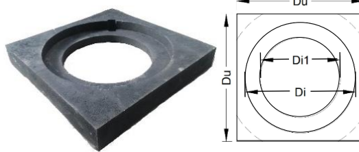
Firkantkarm til Ø315 mm dæksel
