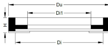
Dæksel m/ karm Ø600 / Ø800 mm består af en topning med fals og et dæksel
