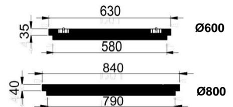
Ø600 / Ø800 karm
