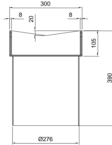
HUGOLINE Ø280
